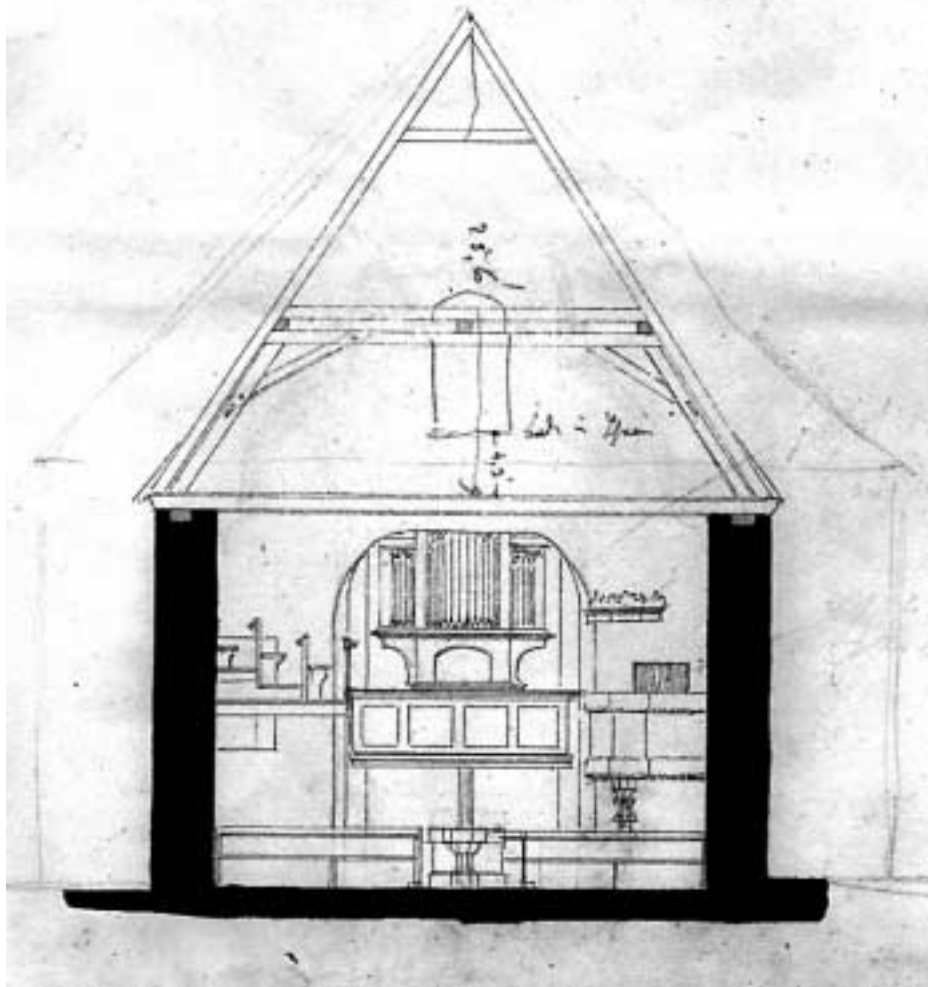
Alte Kirche (1860), Querschnitt gegen den Chor
